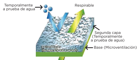
ESTRUCTURA DEL RECUBRIMIENTO DE PU
